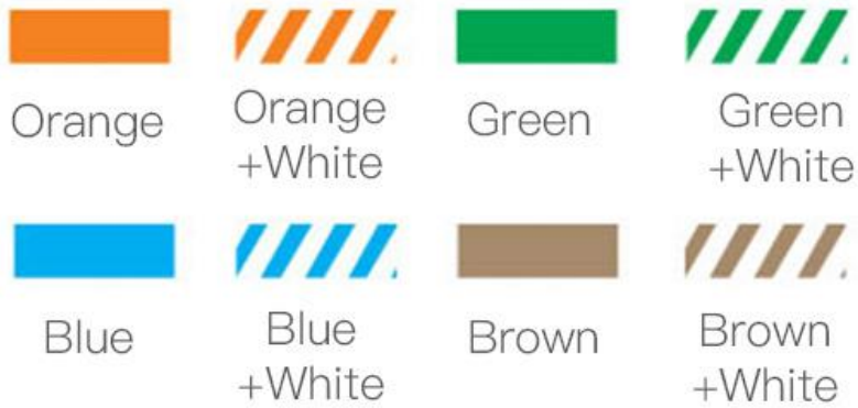
T568A
