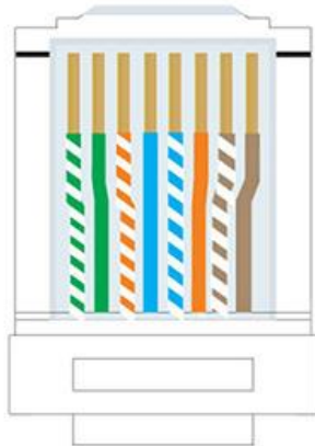
T568A
