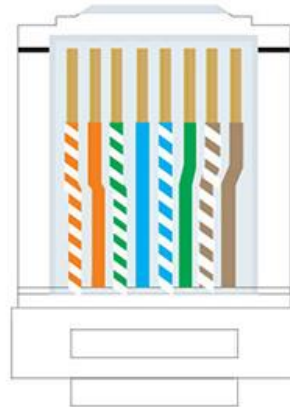
T568B
